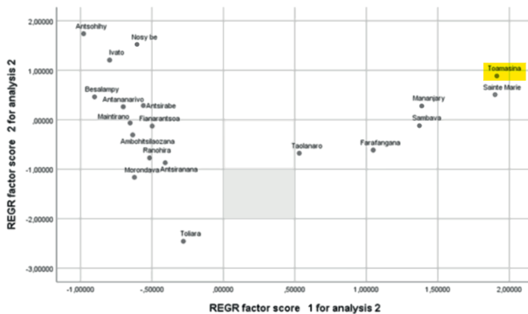
Figure A.1. 1 Répartition des précipitations sur la période 1991- 2020 par station météorologique
