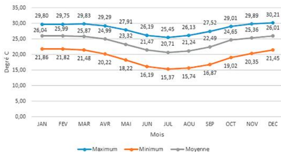
Graphique A.1. 1 Température moyenne par station
